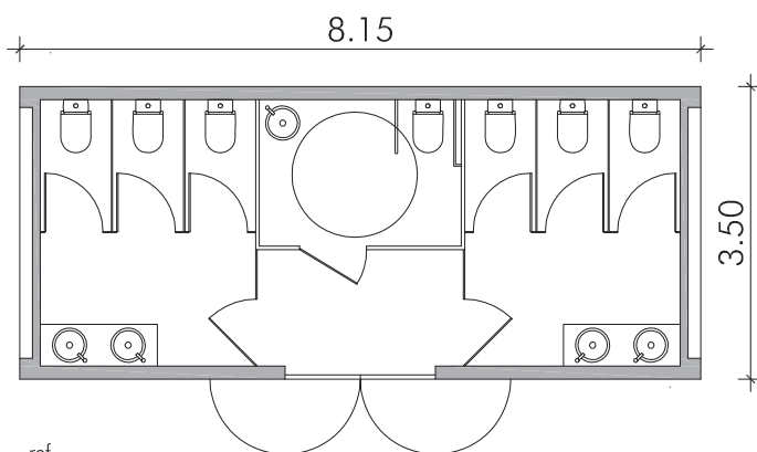
ref. ED01.3581.CX.14Wb Lavabos públics (homes i dones adaptat)
