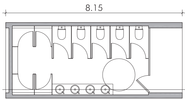
ref. ED01.3581.CX.05W Lavabos i dutxa (adaptat)
