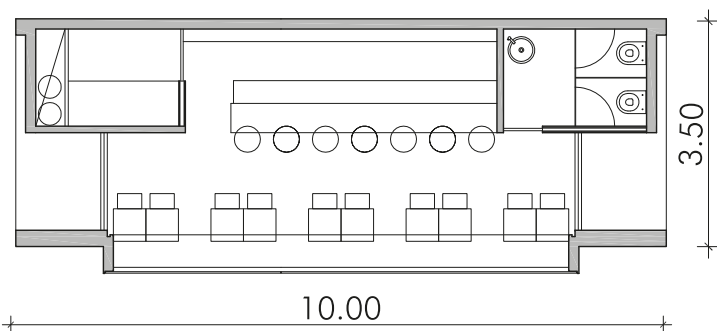
ED01.35100.CX.01B Bar + cuina + banys accés interior
