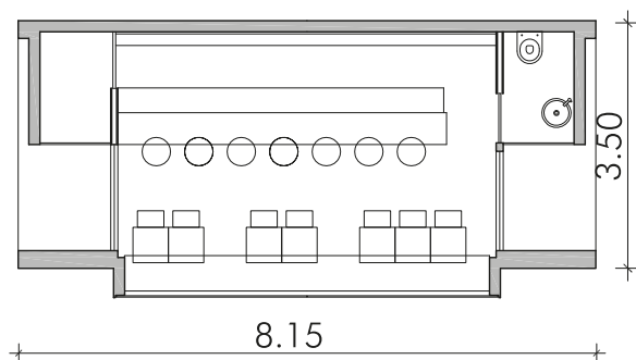
ED01.3581.CX.03B Bar + magatzem + bany accés interior
