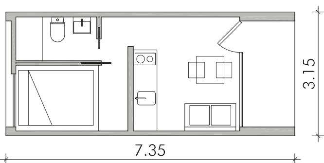
ref. ED01.3173.CX.01C Bungalow/mobile home adossat amb porxada
